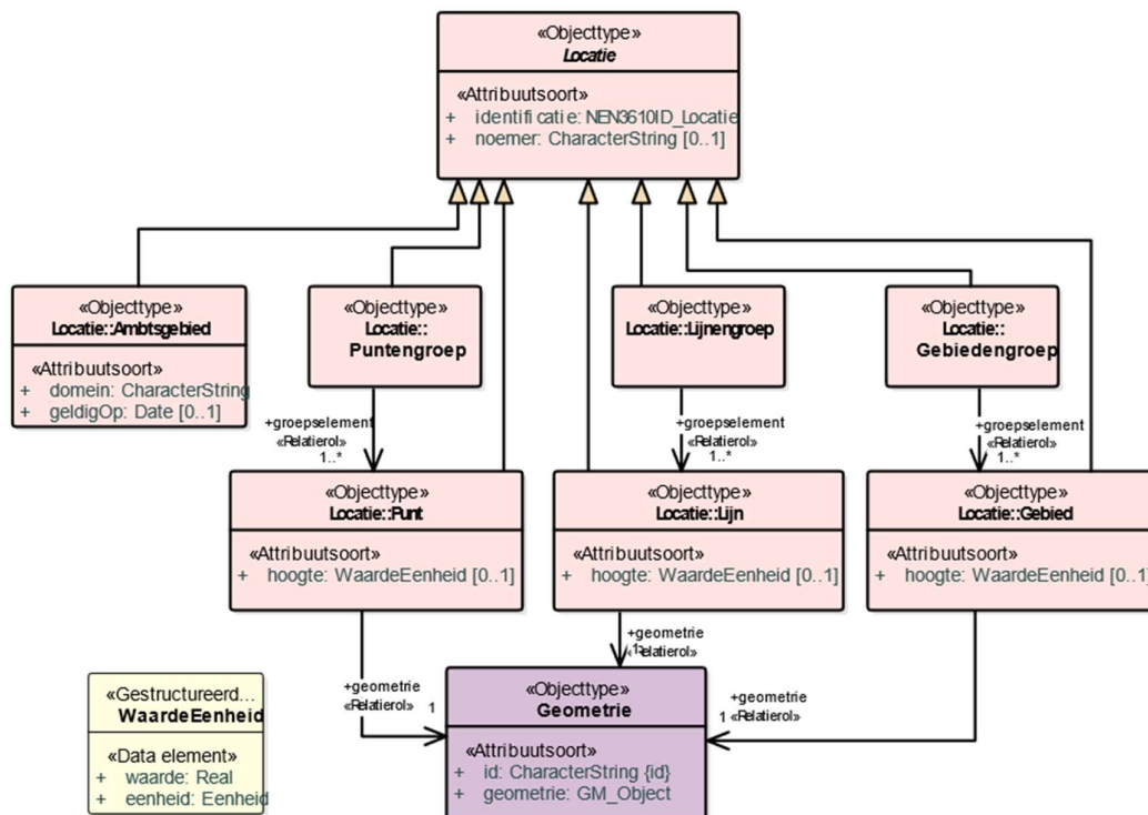
Figuur 11 Uitsnede uit IMOW-diagram voor objecttype Locatie
