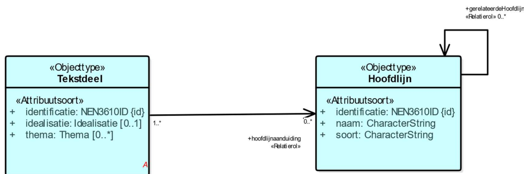
Figuur 10 Uitsnede uit IMOW-diagram voor objecttype Hoofdlijn
